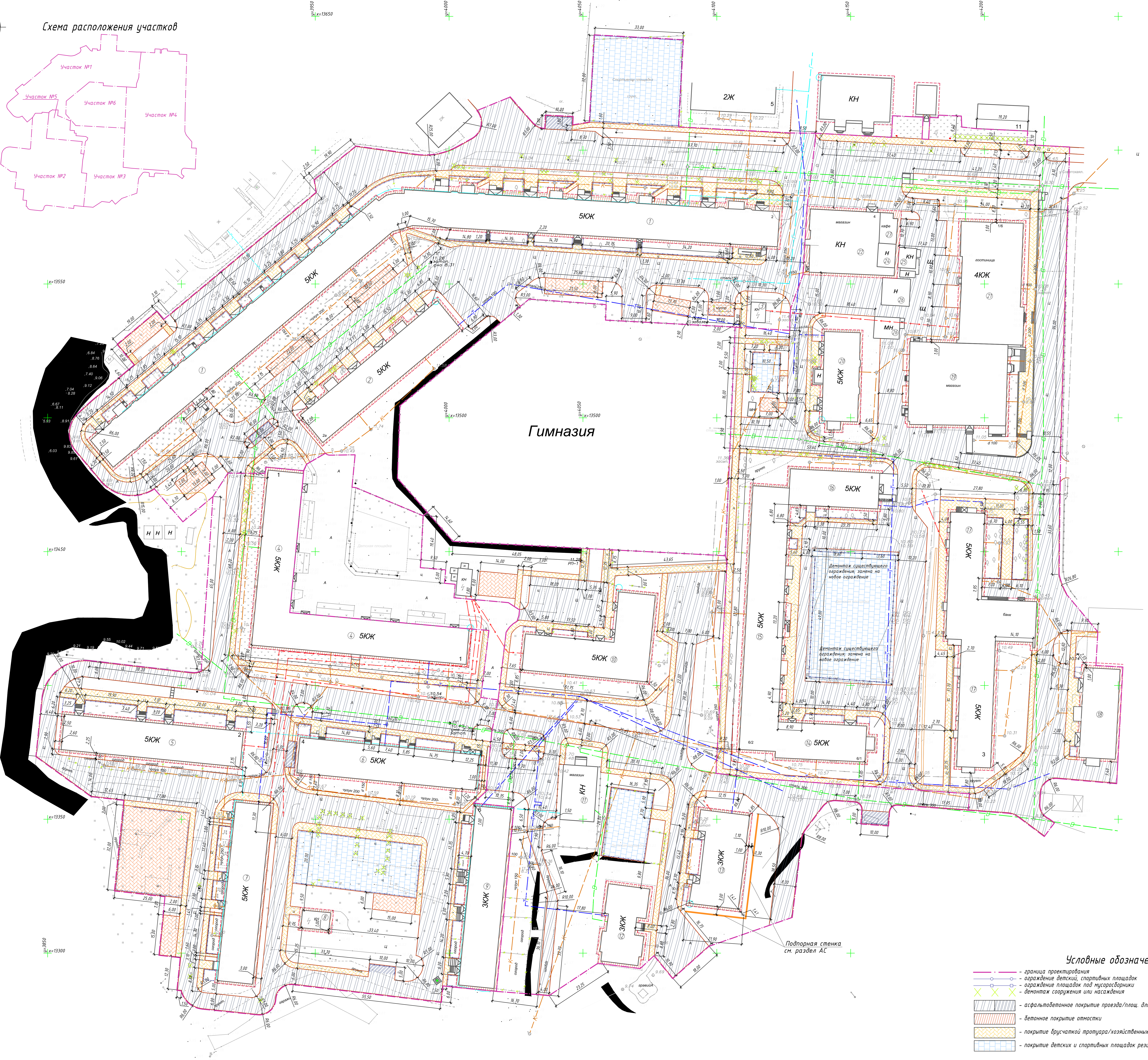
План проездов, тротуаров, дорожек и площадок
