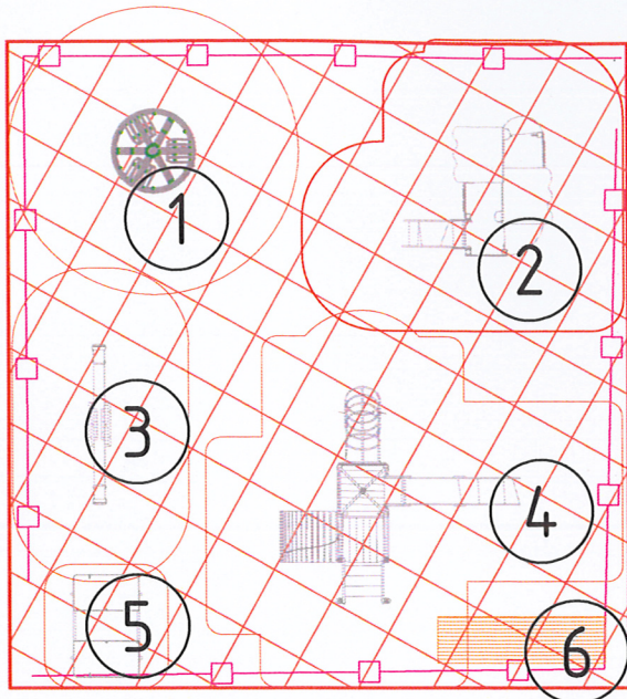
1. 004194 – Карусель с рулем Производитель: "Ксил" Габаритные размеры: D=1640 мм, Н=715 мм, Н площадки=80 мм
